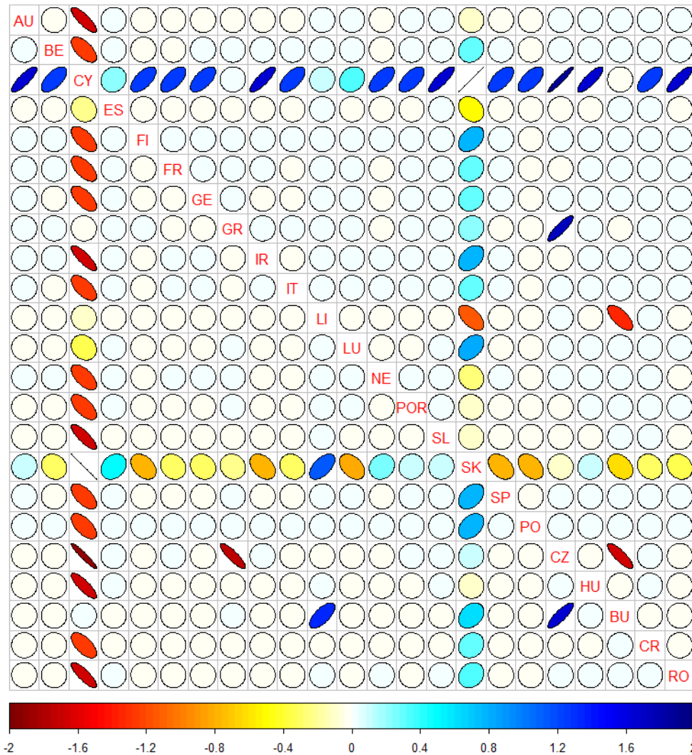
Figura 32 Avans-întârziere ( lead-lag )
